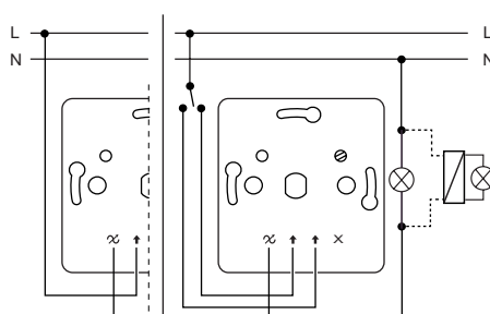
Izmjenična sklopka – EPH66001xx
