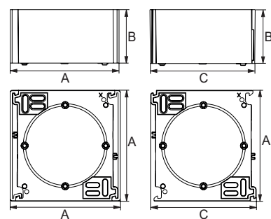
Nadžbukne kutije (mm)
