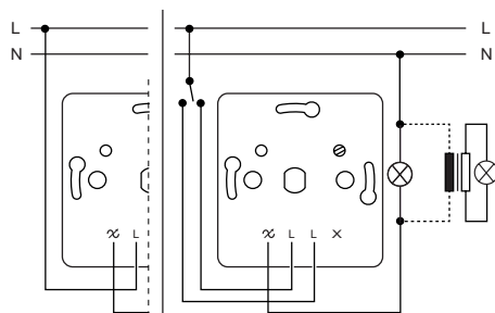
Izmjenična sklopka – EPH64001xx - EPH65001xx
